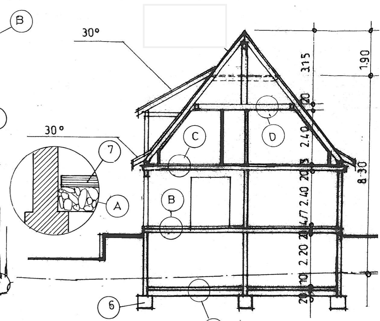
COUPE VERTICALE AA
